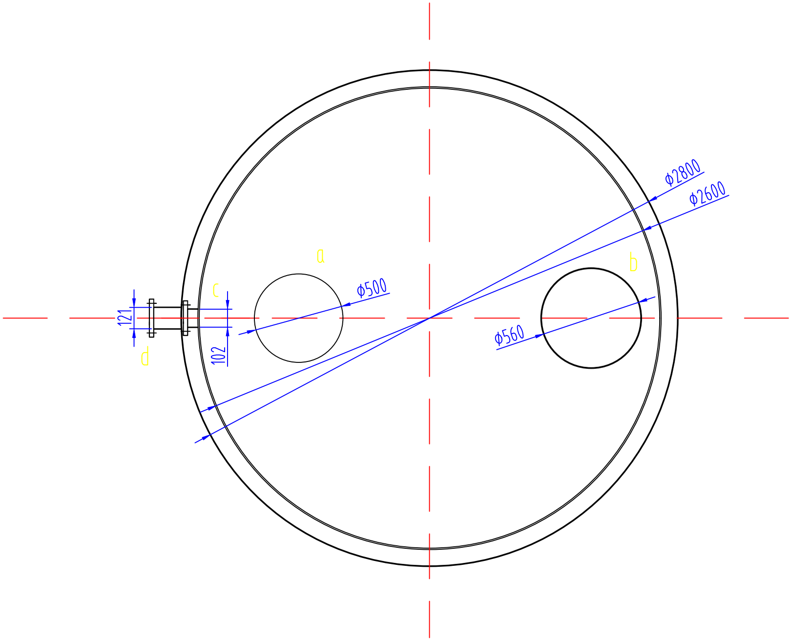
A向俯视图（仅筒体）
